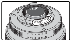
Prozessorgesteuerte Objektive sind an den elektrischen Kontakten zu erkennen.
