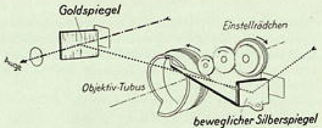
Abb. 24. Schematische Darstellung der automatischen Einstellung der Contax
