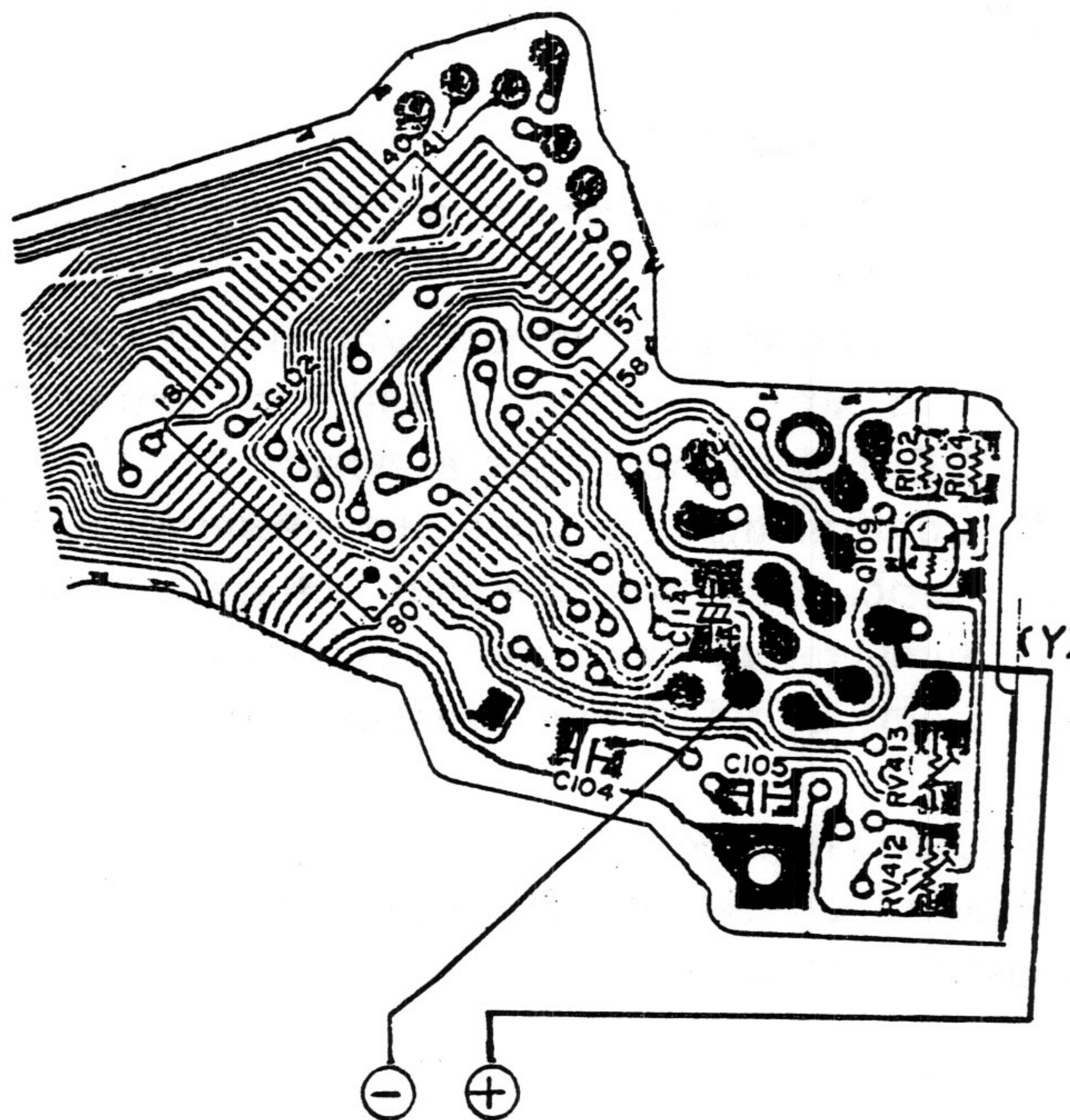
Digital voltmeter
