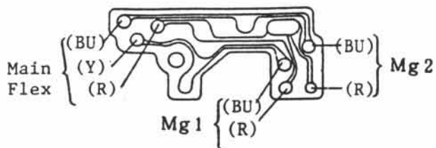
(22) Wiring
