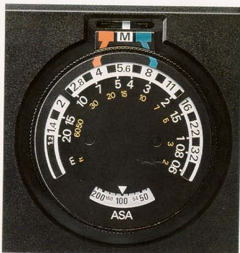
Belichtungsrechenscheibe
