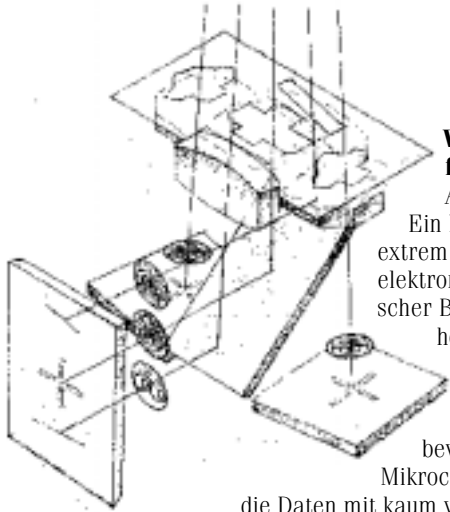
Autofokus-Modul Multi-CAM1300 ① CCD-Kreuz-Sensor für linkes Meßfeld ② CCD-Sensor für oberes Meßfeld ③ CCD-Kreuz-Sensor für mittleres Meßfeld ④ CCD-Sensor für unteres Meßfeld ⑤ CCD-Kreuz-Sensor für rechtes Meßfeld
