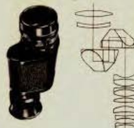
ZEISS-Fernrohrvorsatz 8x30 B Bildwinkel 6°
