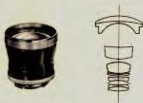
PRO-TESSAR 1:3,2/35 mm Bildwinkel 60°
