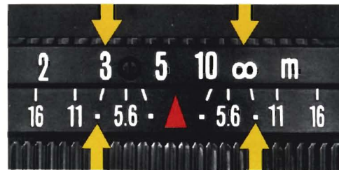
Abb. 3 Entfernungsskala und Schärfentiefering. Bei Blende 8 z. B. von 3 m bis Unendlich.
