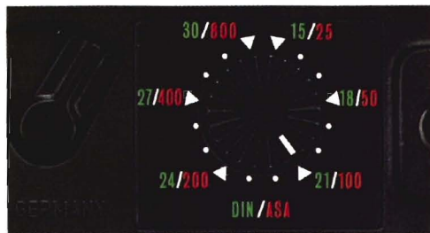
Abb. 7 Die Filmempfindlichkeitsskala ist auf der Unterseite der Minox 35 GL.
