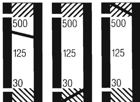
Abb. 5 Links: Die Verschlusszeit wird ca. 1/300 Sekunde betragen. Mitte: Langzeitwarnung (Zeiger im schraffierten Feld unterhalb der 1/30 Sekunde). Rechts: Überbelichtungswarnung (Zeiger im schraffierten Feld oberhalb der 1/500 Sekunde).
