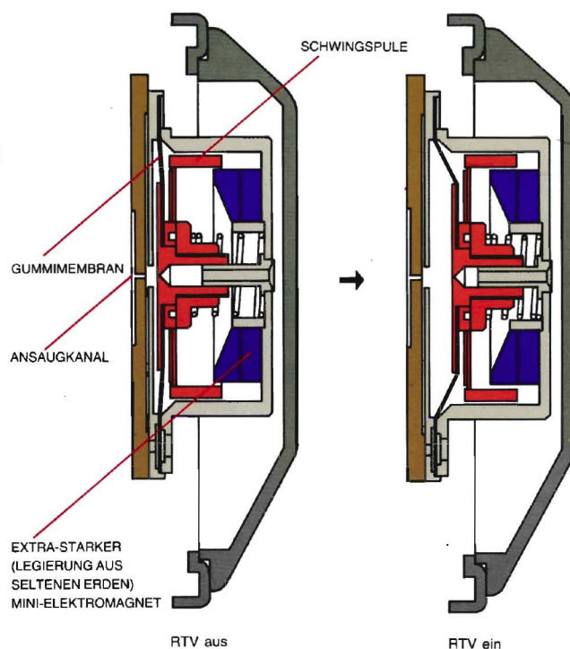
RTV SCHNITTZEICHNUNG
