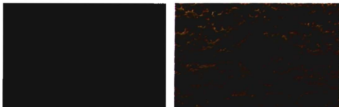
Mikrofotografischer (200x) Vergleich der Oberflächenfestigkeit einer Feinkeramik- (links) und Aluminium- (rechts) Andruckplatte nach dem Aufschlag einer Diamantspitze mit einer Kraft von 1 kg.
