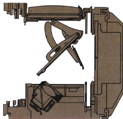
Schnittbild des Spiegelkastens
