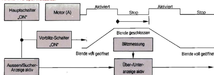
Vorblitz-TTL-Spot-Meßablauf
