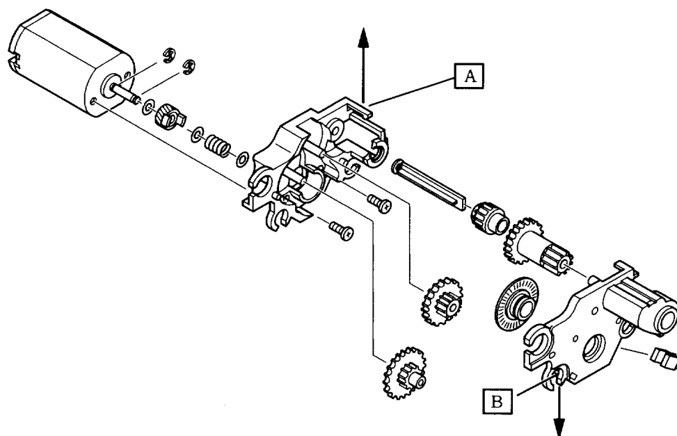
AF base plate unit
